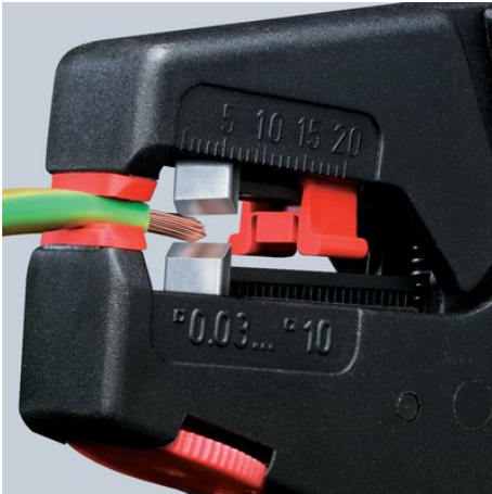
12 40 200: Pelado preciso sin dañar el cable conductor
